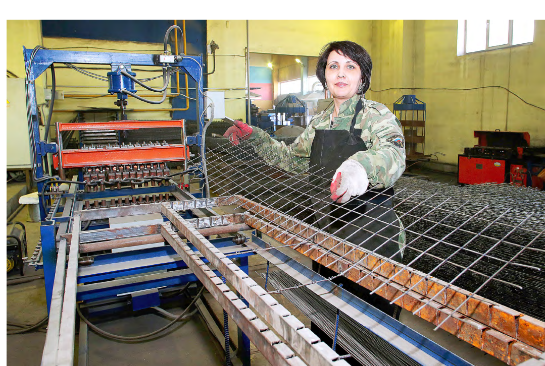
Цех металлоизделий. Участок производства кладочной сетки и арматурных каркасов. Производство кладочной сетки на машине контактной сварки (МТК 650УХЛ-4)
