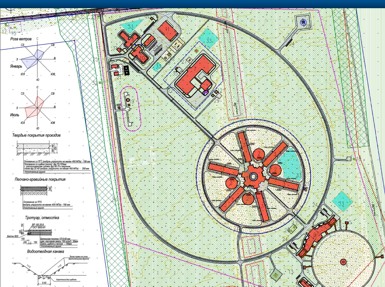
Мастер-план участка
